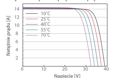
Krzywa natężenie prądu - napięcie
